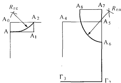
Рис. 6.2. Схема построения горловины спинки и перада
