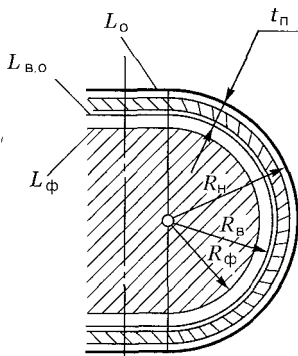
Рис. 5.10. Определение P_n расчетным способом
