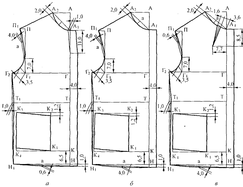
Рис. 14.3. Схема построения детали полочки мужской куртки
