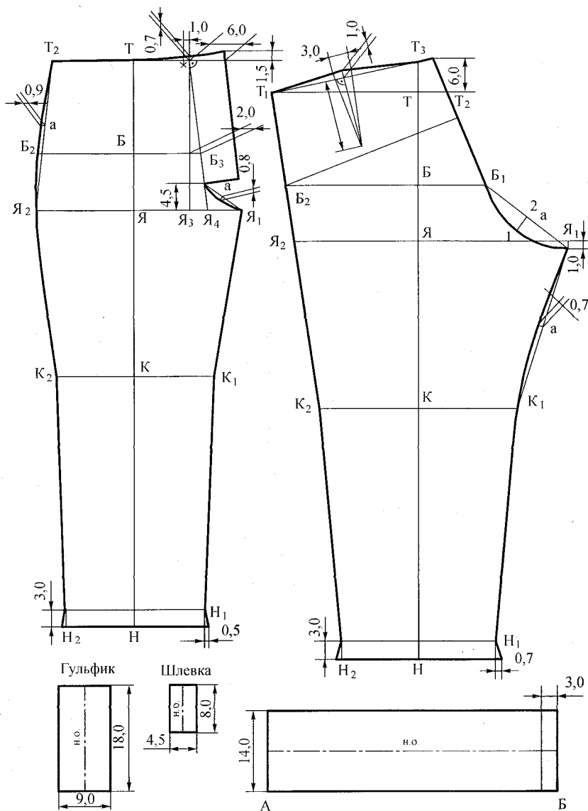
Рис. 14.6. Схема построения чертежа передней и задней половинок и пояса мужских брюк 1-й группы
