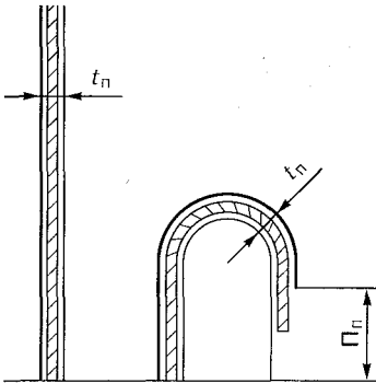
Рис. 5.9. Определение P_n муляжным способом
